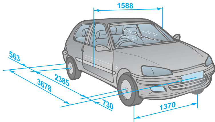
3 door
